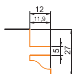
profil poprzeczny
