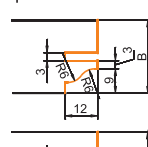
profile wzdłużne
