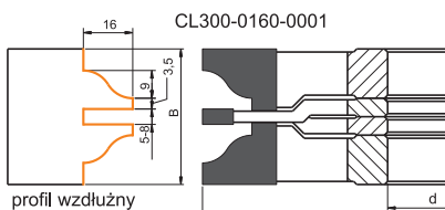
profil wzdłużny
