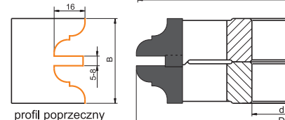
profil poprzeczny
