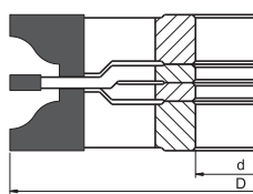
profil wzdłużny
