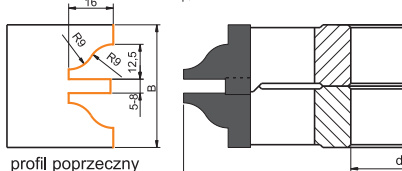
profil poprzeczny
