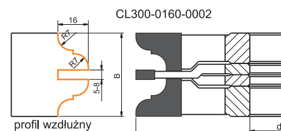
profil wzdłużny
