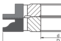
profile wzdłużne
